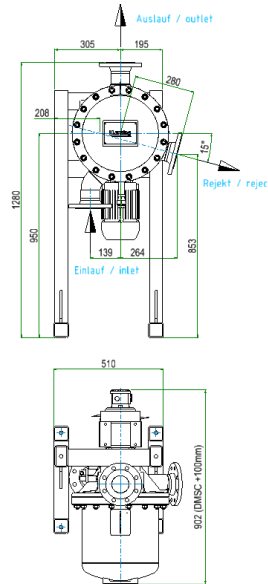
Dimensions OptiFil-M-250-0180
